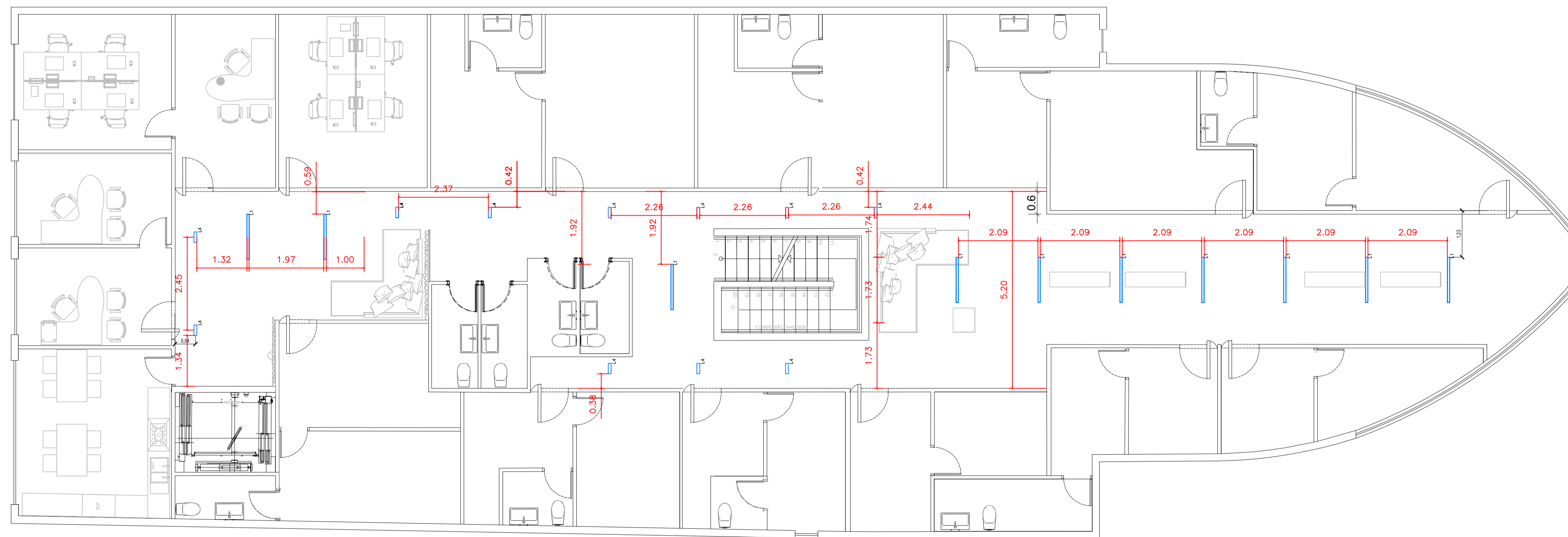
Planta de elétrica . pontos elétricos- 1 PAVIMENTO Escala 1/75
