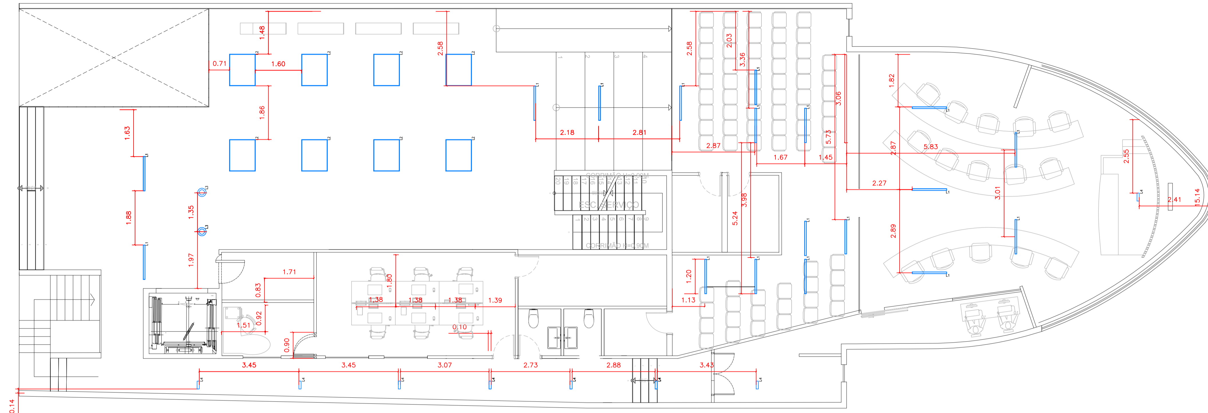
Planta de elétrica . pontos elétricos- TÉRREO Escala 1/75
